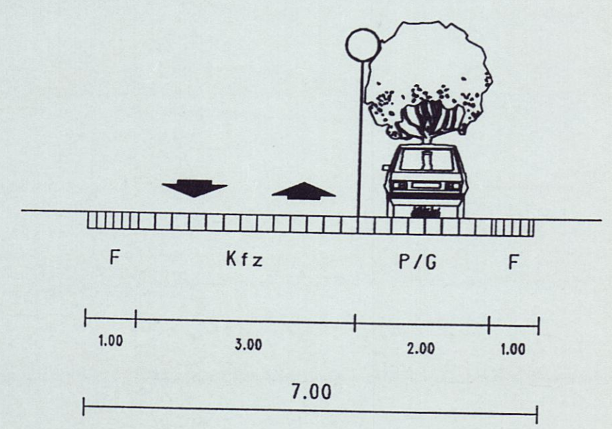
Schnitt A - A SYSTEMSCHNITT Straßenraum
